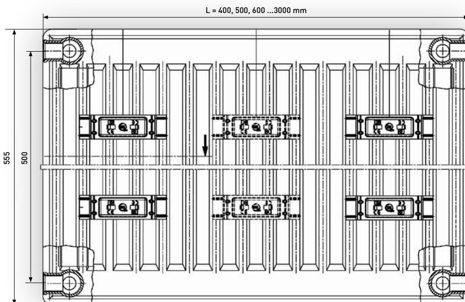
Renovierungsheizkörper Typ 22
