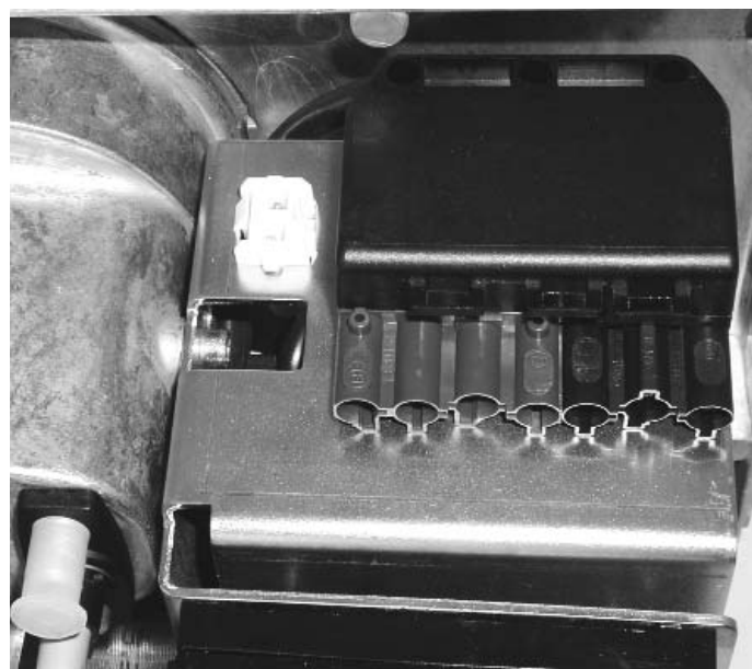
Abbildung 32 - Netzanschluß – Eurostecker Figure 32 - Power connection – Euro-plug - Prise Européenne raccordement sur secteur
