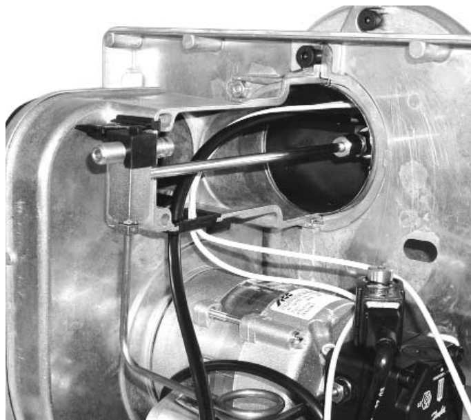
Abbildung 30 - Ausbau des Düsenstocks Figure 30 - Disassembly of the nozzle - Démontage de ligne gicleur
