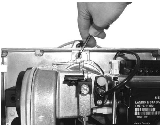
Abbildung 25 - Lösen der Service-Schraube Figure 25 - Loosening of the service screw - Dévisser la vis de service
