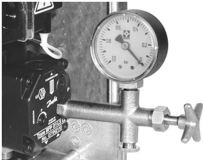
Abbildung 31 - Vakuummessung Figure 31 - Vacuum measurement - Vacuum mesurage
