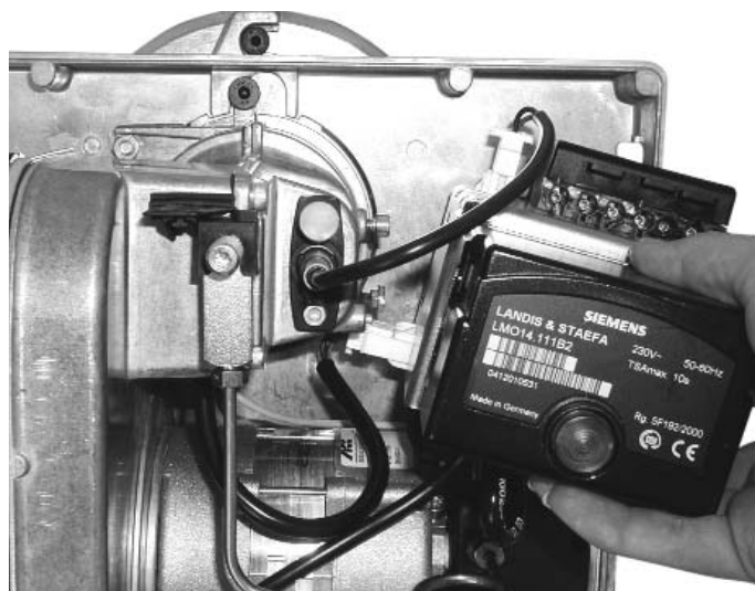
Abbildung 28 - Steuereinheit abgenommen Figure 28 - Control unit removed - Organe de commande retiré
