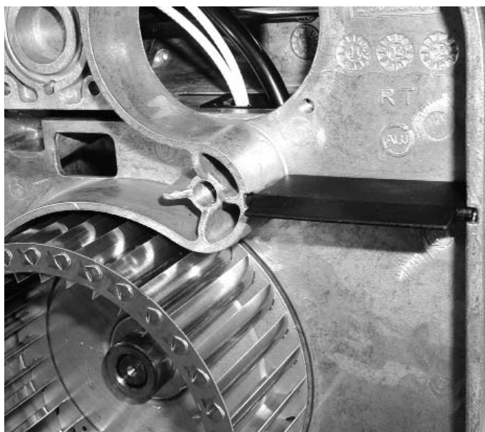
Abbildung 26 - Einbaulage der Luftklappe Figure 26 - Installation position of the air flap - Position de montage du clapet d'air
